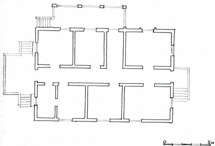
7. Plan (relevéle și planurile întocmite de arh. N. Goga)
