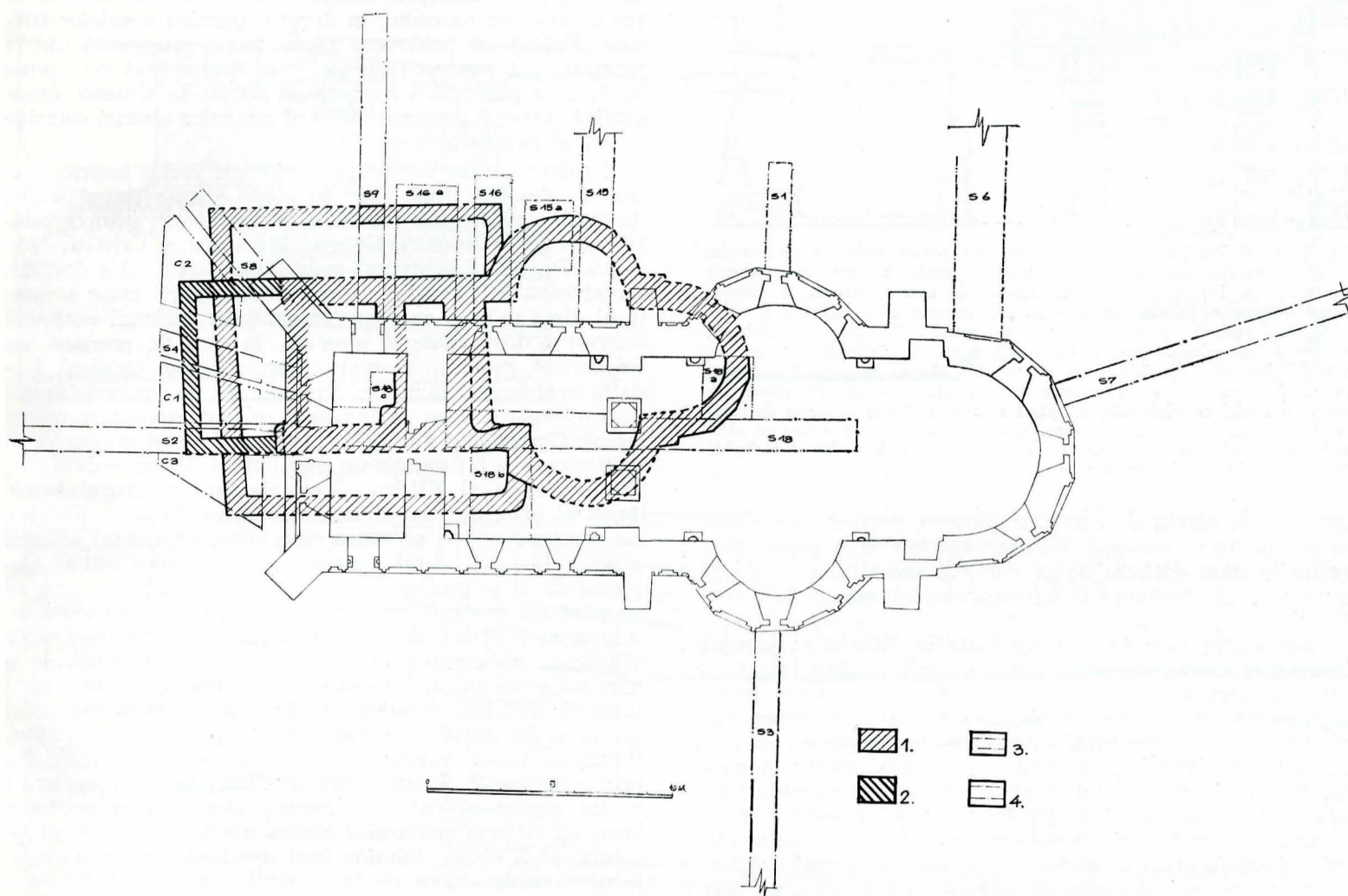
Fig. 1. Planul săpăturilor: 1. Fundațiile bisericii de la sfârșitul sec. XVI. 2. Fundațiile exonartexutului adăugat. 3. Săpături 1970—1973. 4. Săpături 1969.
