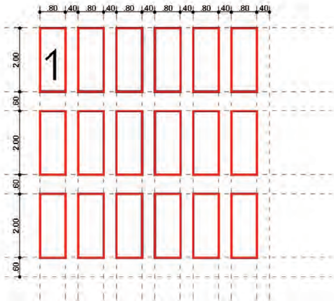
SCHEMA DE BAZA
