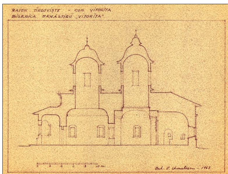
Fig. 14 – Secțiune biserică de arh. Violeta Cherulescu, 1963, arhiva I.N.P.
