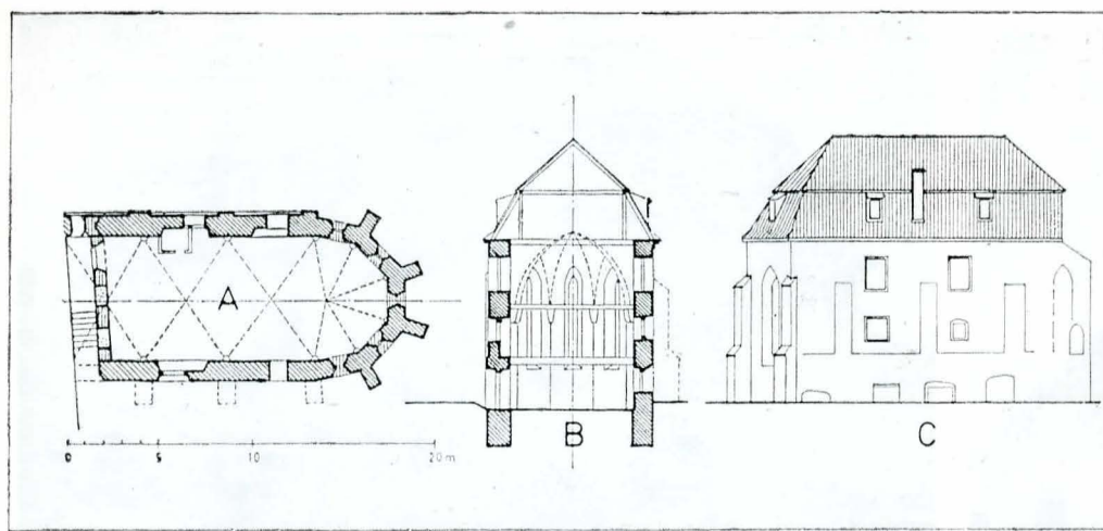
Fig. 2. Releveul corului bisericii Mănăstirii călugărițe or franciscane. Situația mai 1987. A — Plan, la nivelul parterului cu indicarea elementelor originare gotice, hașurate la 45°; B — Secțiune transversală spre est, C — Fațada nord cu indicarea pilaștrilor și a golului de fereastră gotică spre vest.
