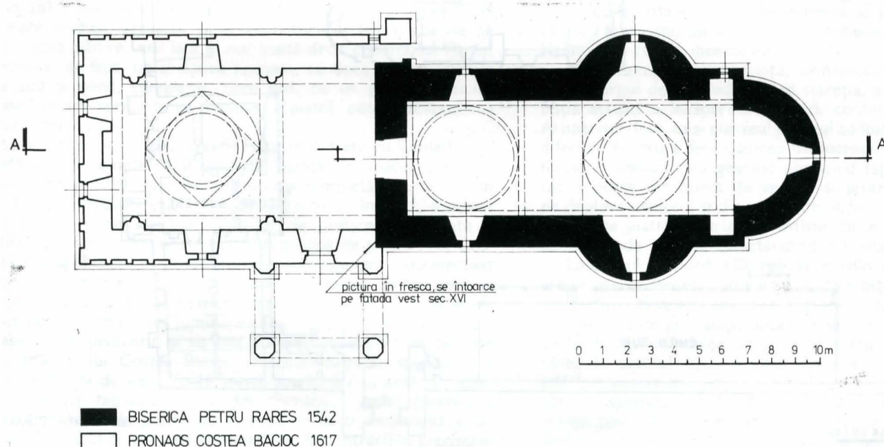
Biserică Plan 1:100
