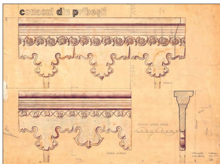
Fig. 12. Detalii ale foișorului de est - Releveu, 1950 (autori: stud. arh. C. Frumuzache, I. Antonescu, Ivonne Goldenberg, Raul Sorin)
