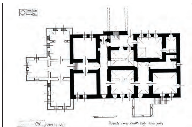
Fig. 4. Plan parter - Releveu cca 1944 (autor: arh. Ștefan Balș)
