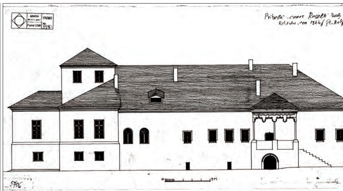
Fig. 3. Fațada principală - Releveu, cca 1944 (autor: arh. Ștefan Balș)
