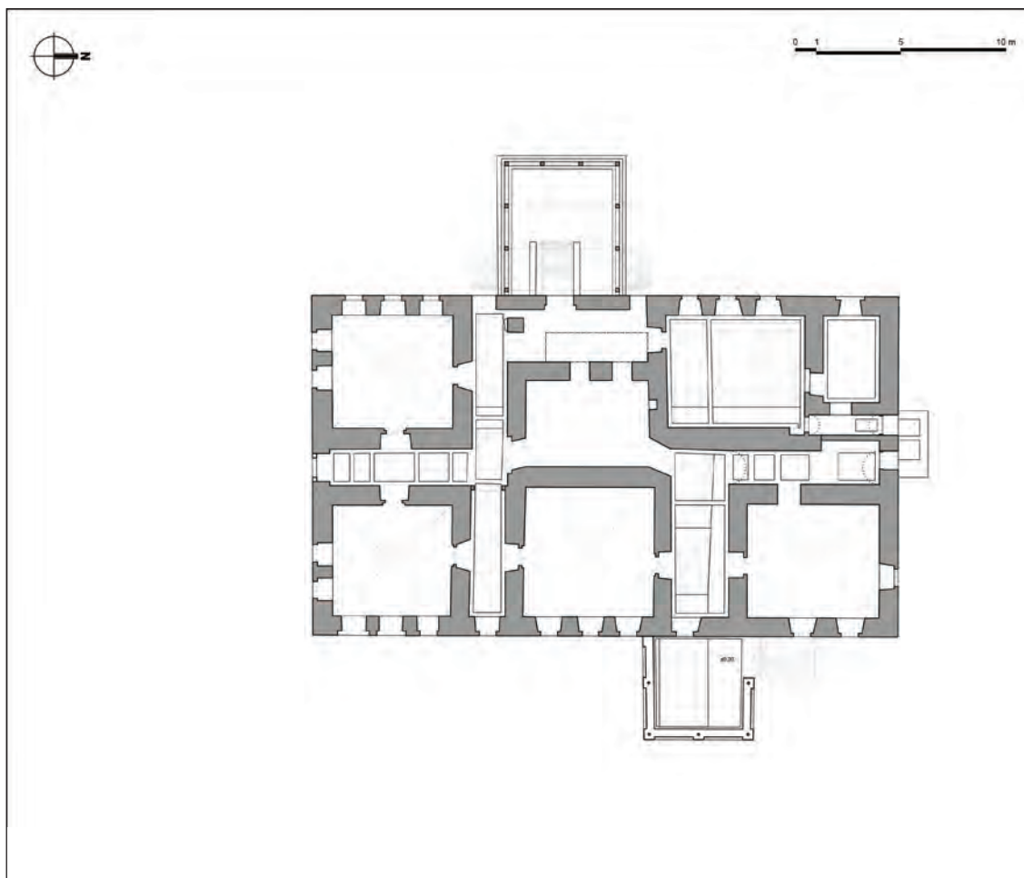
Fig. 19. Plan parter – după Releveu, 2016 (șef proiect: arh. Petru Mortu, relevat și desenat: Alexandru Găgiu, Alexandra Teodor)
