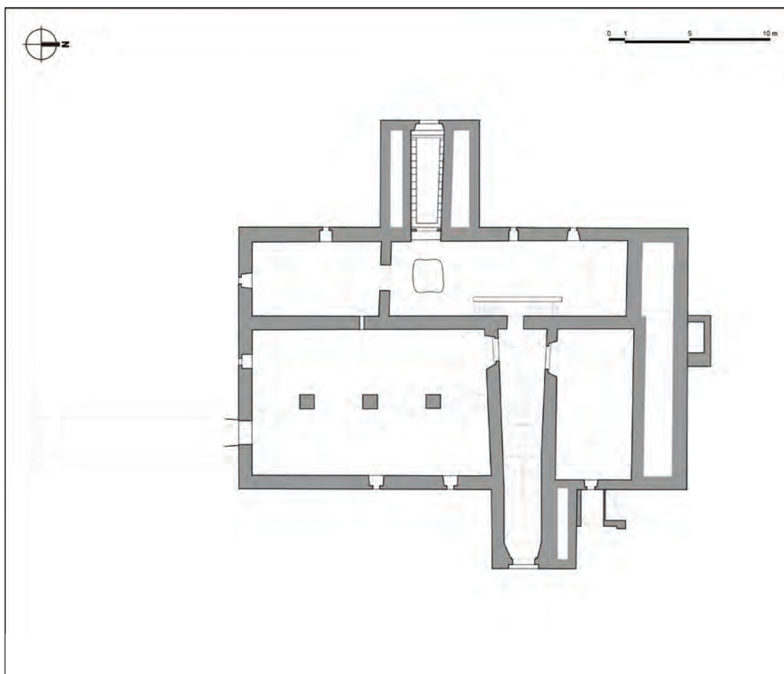
Fig. 18. Plan subsol – după Releveu, 2016 (șef proiect: arh. Petru Mortu, relevat și desenat: Alexandru Găgiu, Alexandra Teodor)
