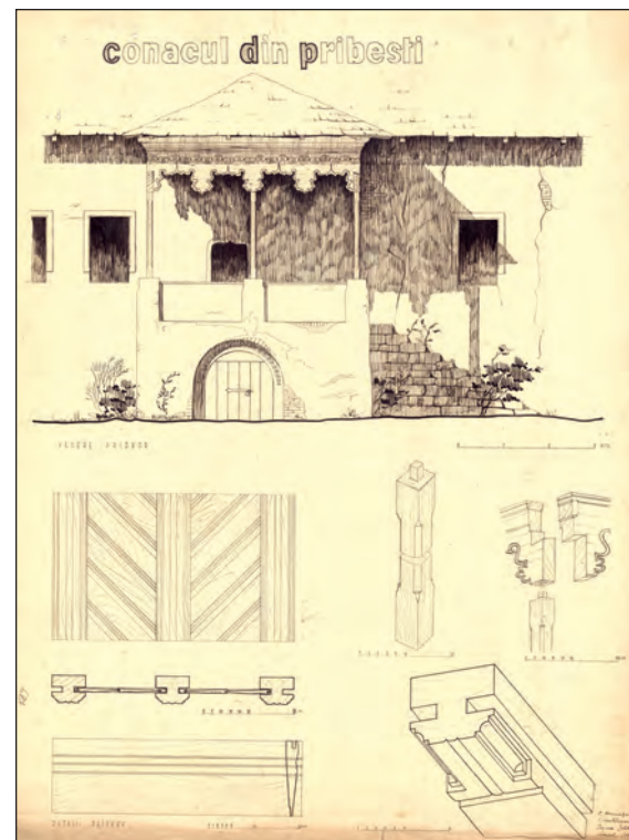
Fig. 11. Fațadă și detalii ale foișorului de est - Releveu, 1950 (autori: stud. arh. C. Frumuzache, I. Antonescu, Ivonne Goldenberg, Raul Sorin)
