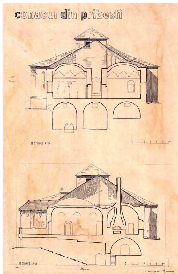
Fig. 14. Secțiuni transversale - Releveu, 1950 (autori: stud. arh. C. Frumuzache, I. Antonescu, Ivonne Goldenberg, Raul Sorin)
