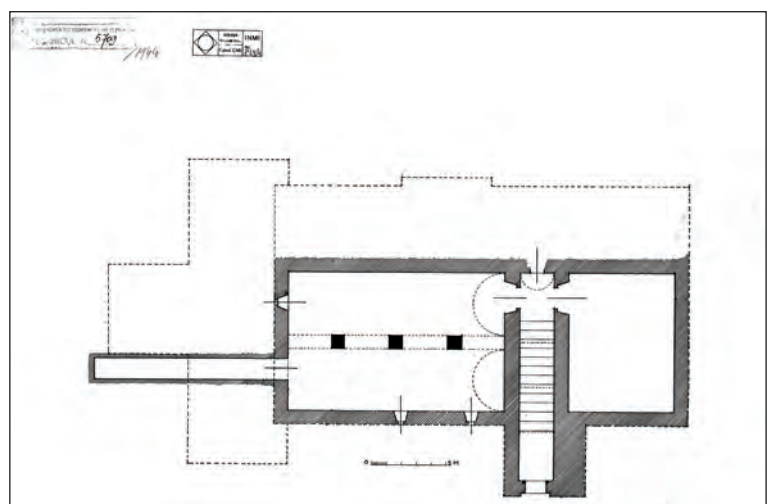
Fig. 5. Plan subsol - Releveu, cca 1944 (autor: arh. Ștefan Balș)
