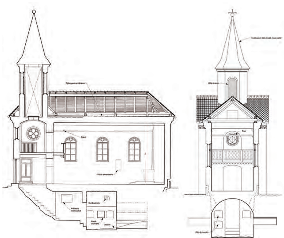
Fig. 13. Capela „Sf. Ecaterina” a fostului cimitir romano-catolic. Secțiune longitudinală și Secțiune transversală. Relevu 2015, arh. Klaus Birthler
