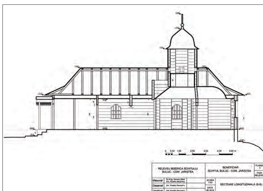
Fig. 6, 7, 8. Relevu, plan și secțiune a bisericii de lemn aparținând Schitului Buluc Planșele relevului desenate de arh. Alexandru Rusete
